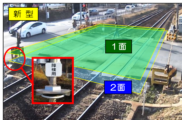
新型障検レーザレーダ式の検知イメージ ・踏切内にいると検知装置が働きます。高さの違う2面で踏切内を検知しております
